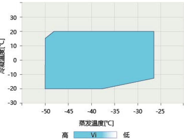
R744制冷剂时压缩机的应用范围
