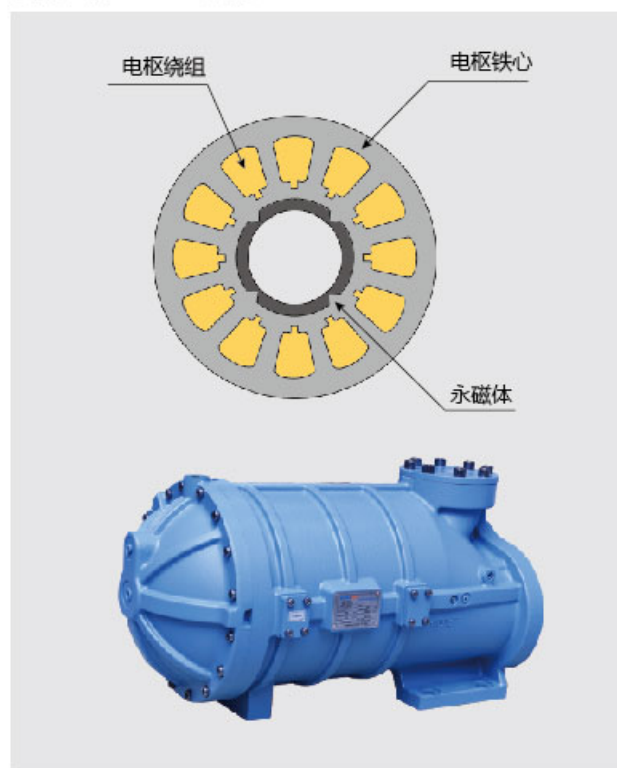
变频永磁同步电机示意图
