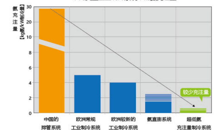
不同类型工业制冷系统中的氨充注量
