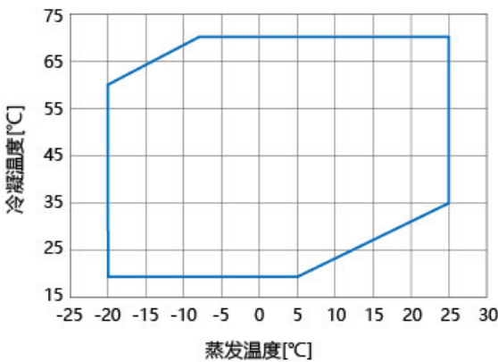
SS5H系列应用范围：R134A
