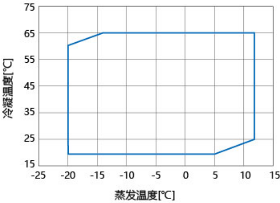
SS5F系列应用范围：R134A
