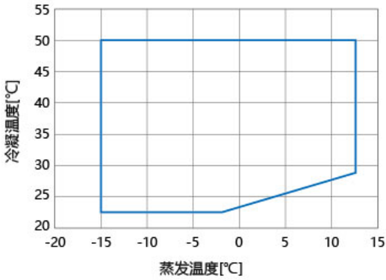
SS5W系列应用范围：R134A
